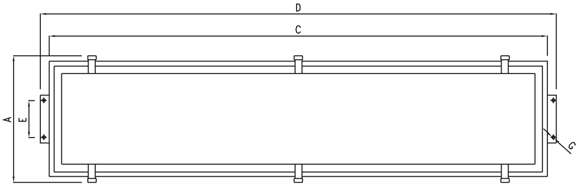
Bovenaanzicht
